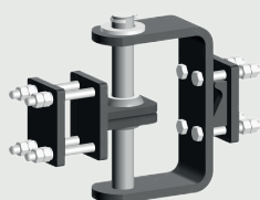
СУС 00.16.000 CB Устройство соединительное
